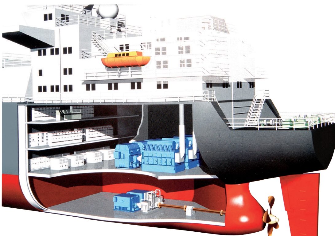
Cámara de máquinas
