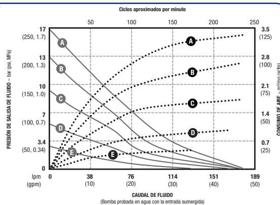
CONFIGURACIÓN DE ALTA PRESIÓN
