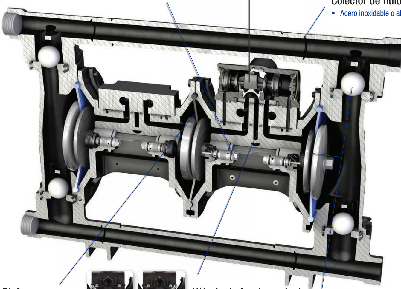
Configuración de baja presión
