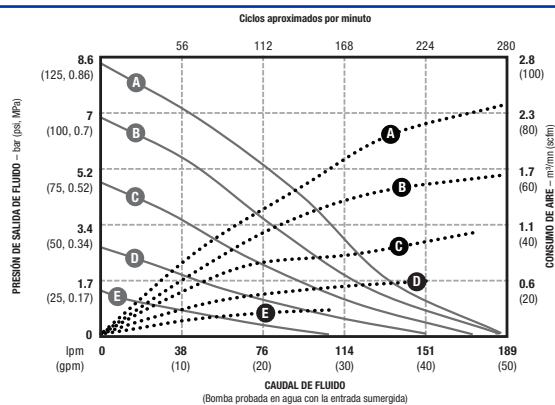
CONFIGURACIÓN DE BAJA PRESIÓN
