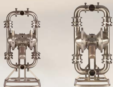
SaniForce 1590 HS 50,8 mm (2 in)
